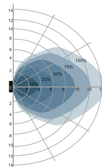
Tunnistusalue seinään asennettaessa (yksikkö: m) Suositeltu asennuskorkeus: 2,5–6 m.
