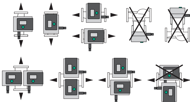
Fig. 3: Toegestane inbouwposities
