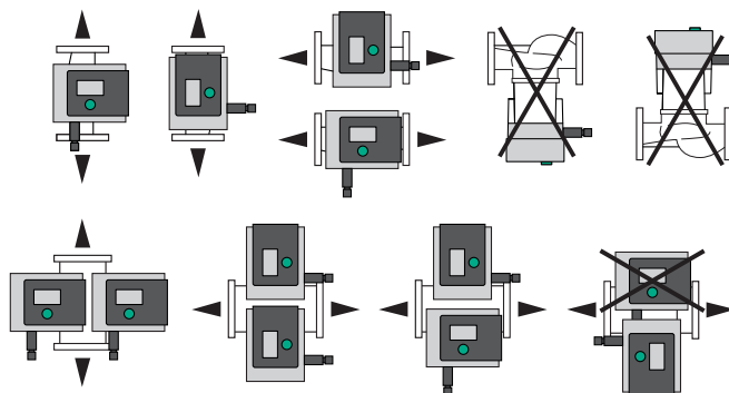
Fig. 10: Megengedett beépítési helyzetek
