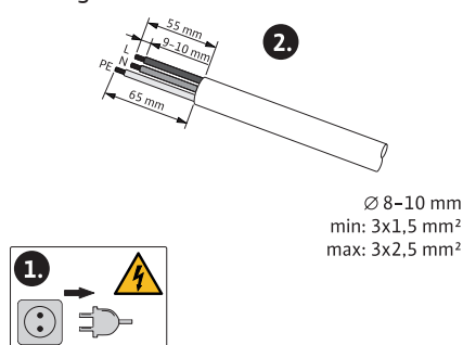
Fig. 21: Aansluiting voorbereiden
