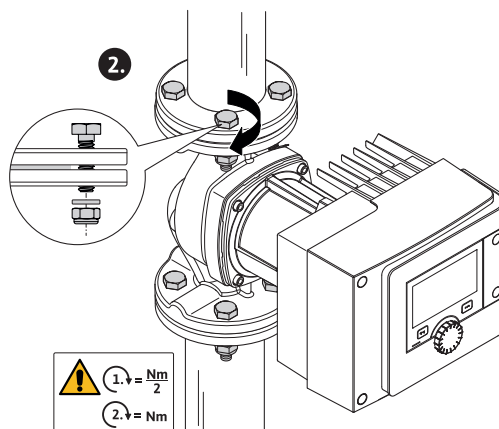
Fig. 16: Montar bomba
