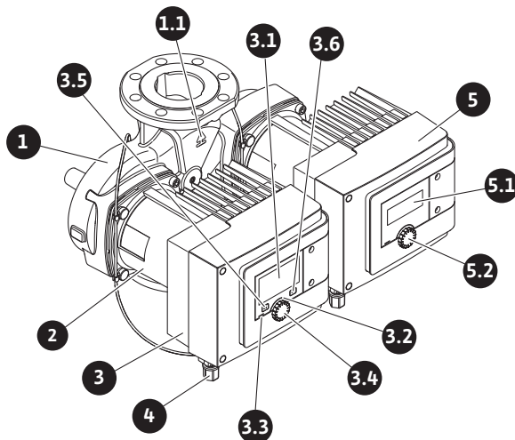
Fig. 2: Pregled dvostruke pumpe
