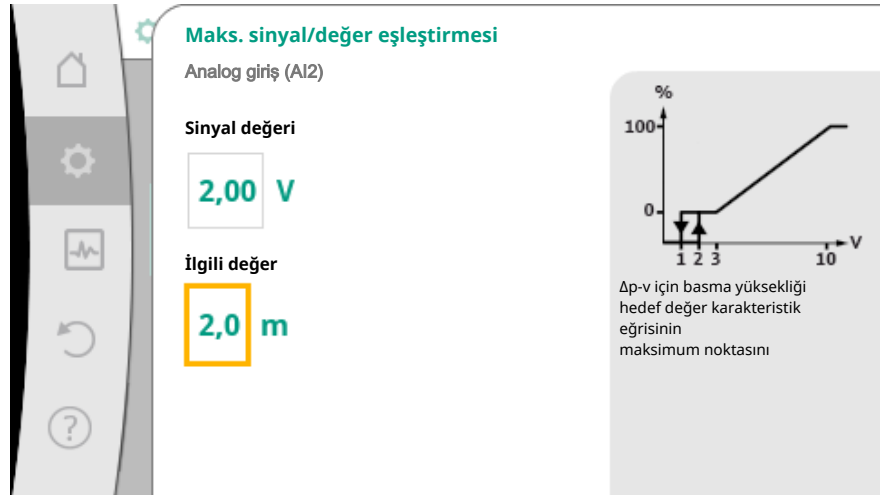
Fig. 76: Maks. sinyal/değer eşleştirmesi
