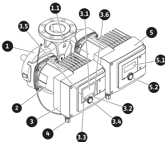
Fig. 2: Pregled dupleks pumpe
