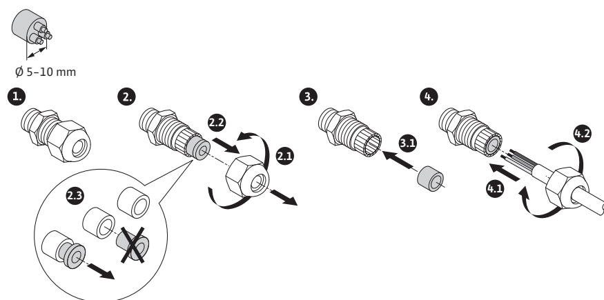
Fig. 22: Kabelskjøt med gjenger Ø 5–10 mm
