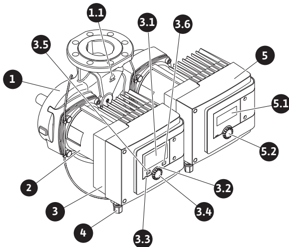
Fig. 2: Sudvejinto siurblio apžvalga
