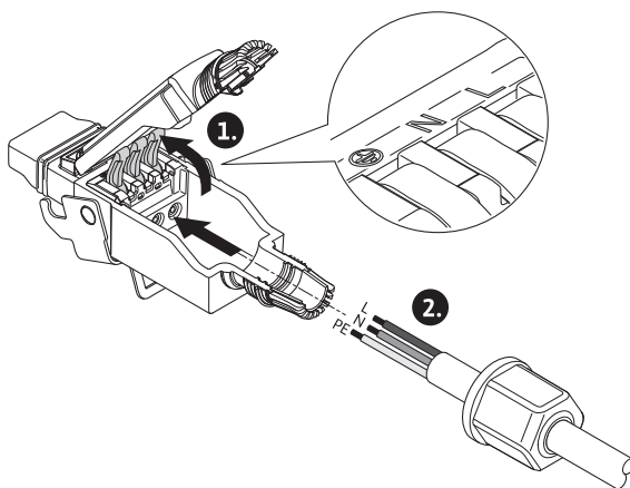
Fig. 26: Kabelio įvedimas
