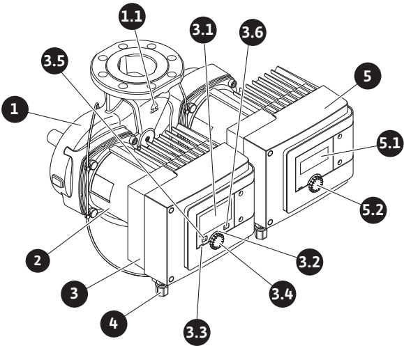
Fig. 2: Vista geral da bomba dupla
