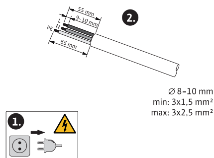
Fig. 24: Förbereda anslutning
