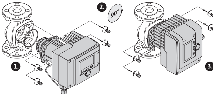
Fig. 19: Otočte motor
