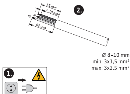
Fig. 24: Sagatavošanās pieslēgšanai
