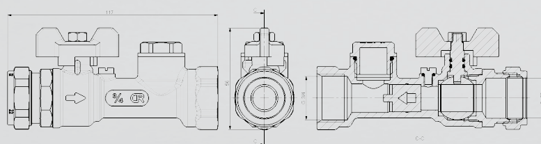
Pumppu/ syöttöventtiili 3/4 sk x 18/22 CU
