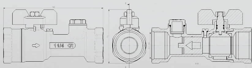
Pumppu/ syöttöventtiili 1 1/4 sk x 1 1/4 sk
