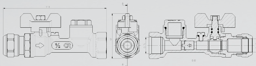
Pumppu/ syöttöventtiili 1/2 sk x 12/15 CU
