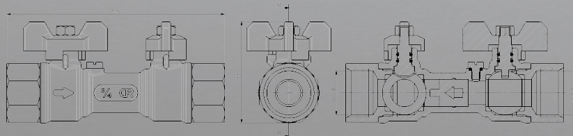
Täyttöventtiili 3/4 sk x 3/4 sk
