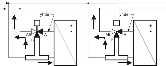
Kuva 3. Ohituskanavalla varustettu kolmitieventtiili
