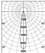
Keskileveä valonjako, 1100 lm
