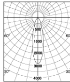
Keskileveä valonjako, 2000 lm
