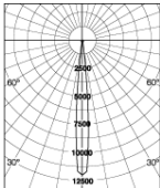
Kapea valonjako, 1100 lm
