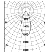
Leveä valonjako, 3000 lm
