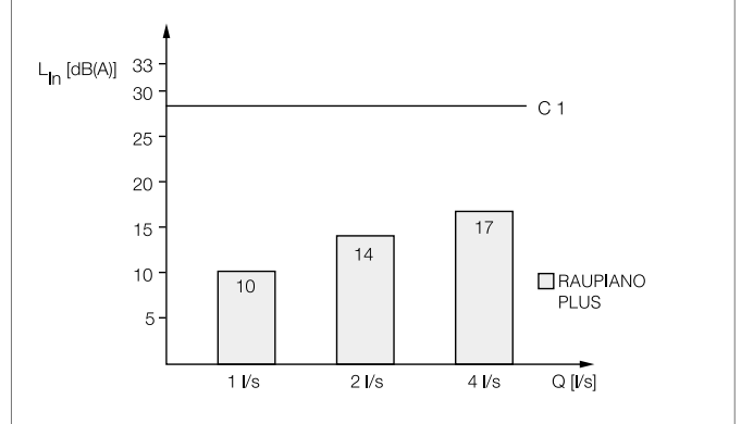
SFS-EN 14366 mukainen testitulos äänenvaimennuksesta eri virtaama-arvoilla
