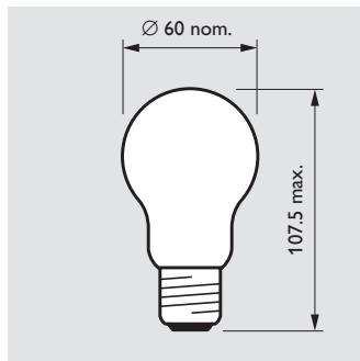
A60 E27
