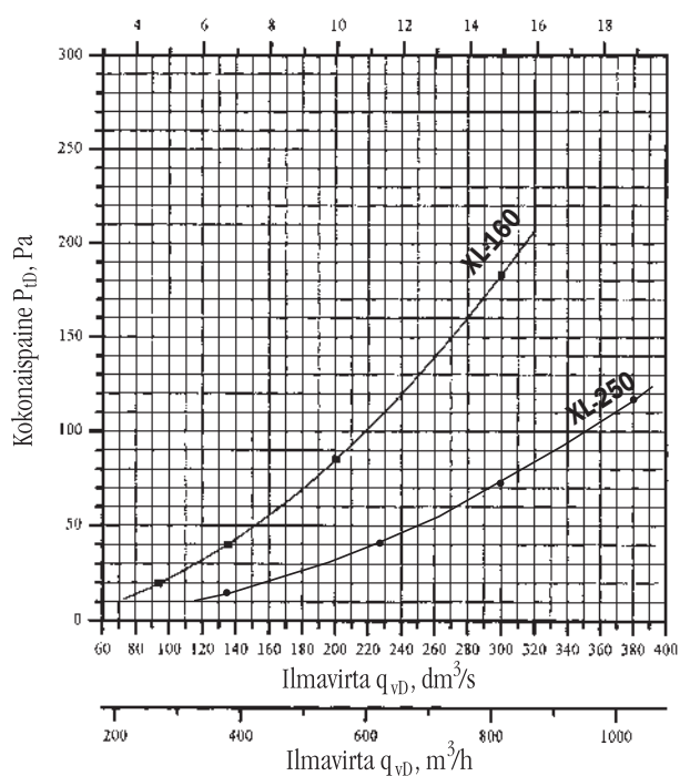
XL-Tiili-pohjalevy
