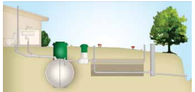
Suodatusputkistopaketti LVI-nro: 3625 430 + 3625 520
