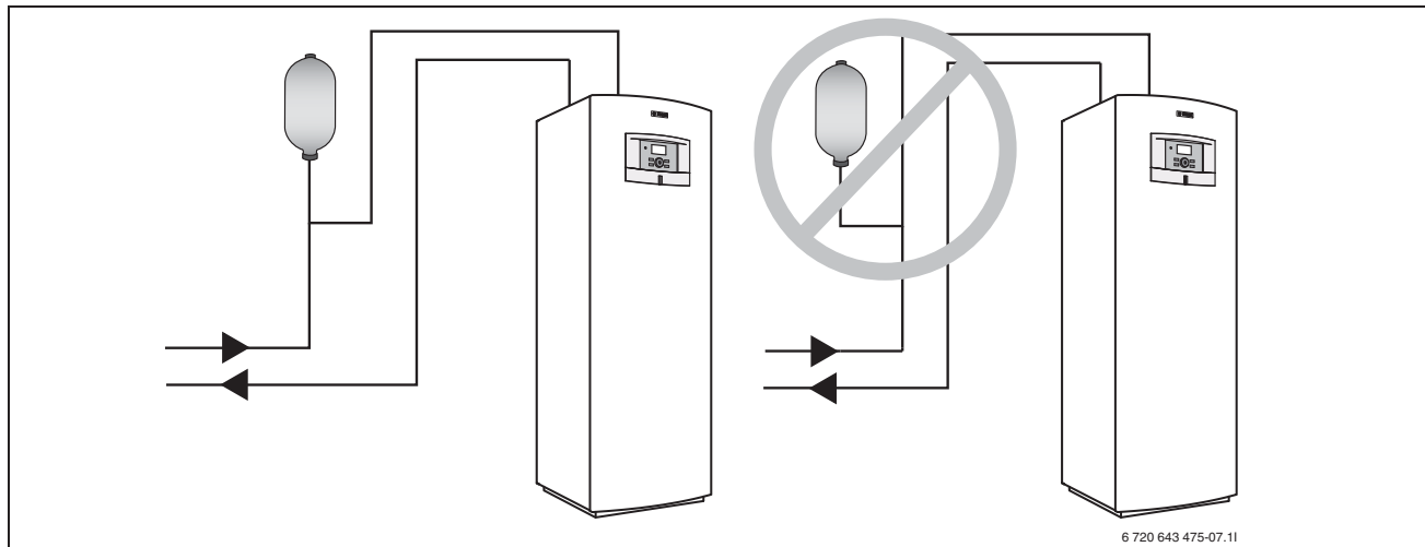
Kuva 18 Paisuntasäiliön asentaminen
