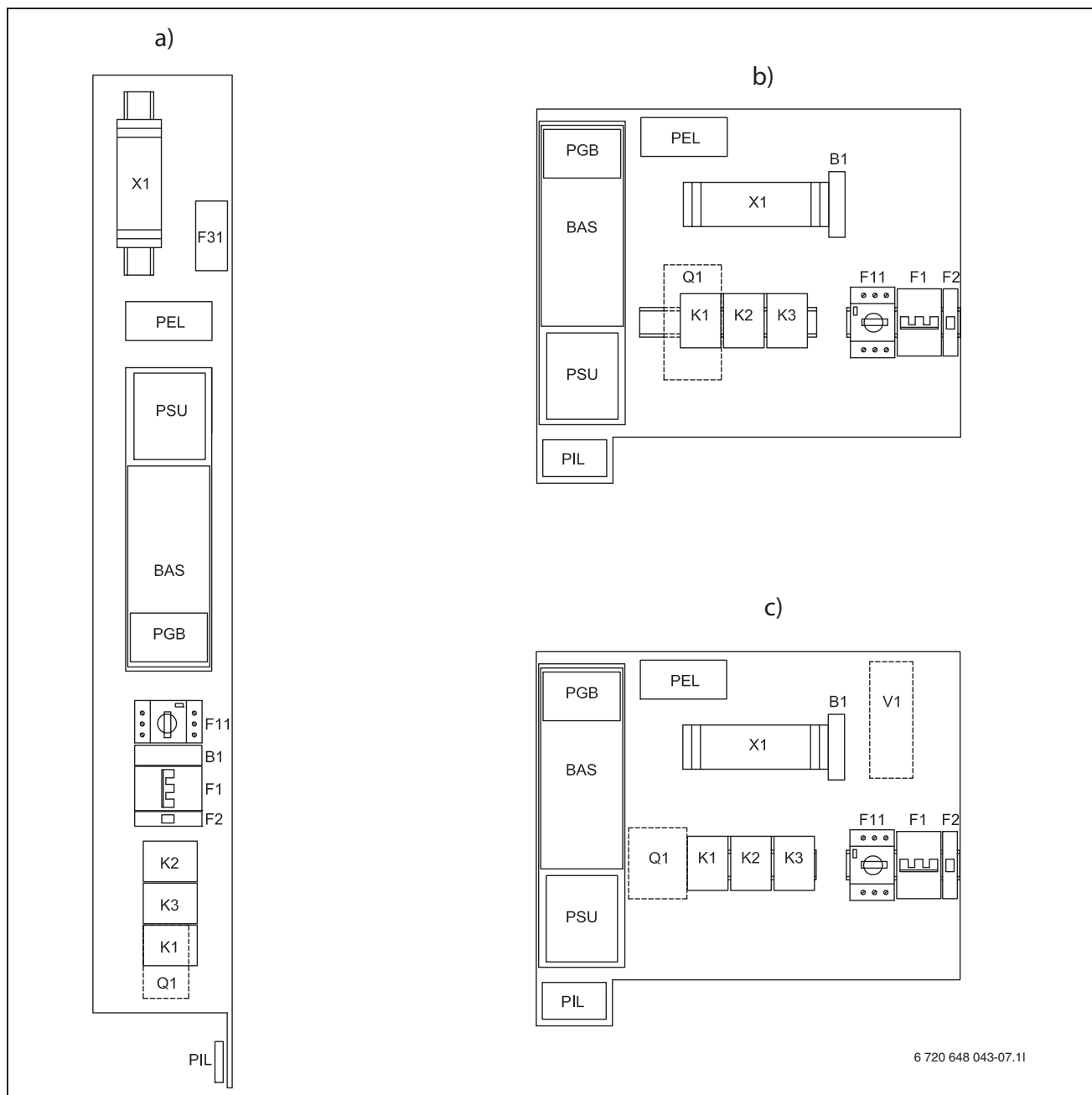
Kuva 38 Piirikorttien yleiskatsaus
