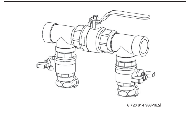
Kuva 23 Täyttösarja 14-17 LW
