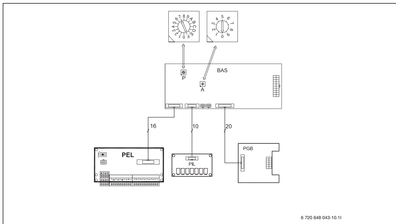
Kuva 40 Piirikortin johdotus
