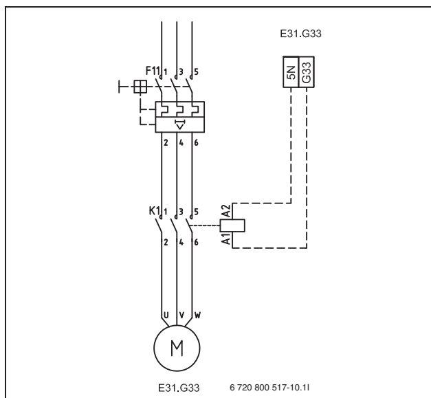
Kuva 45 Pohjavesipumpun liitäntä
