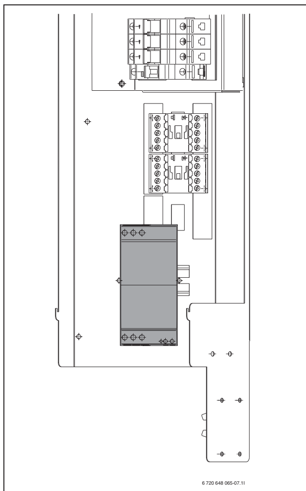
Kuva 32 Pehmökäynnistys asennettuna
