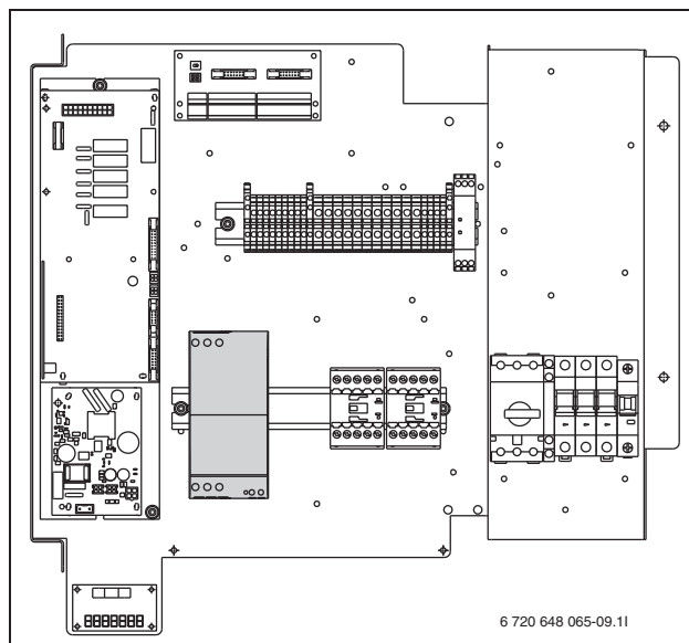
Kuva 34 Pehmökäynnistys asennettuna
