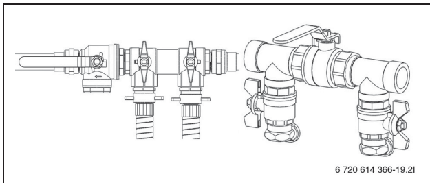
Kuva 25 Täyttösarjat täyttöasennossa
