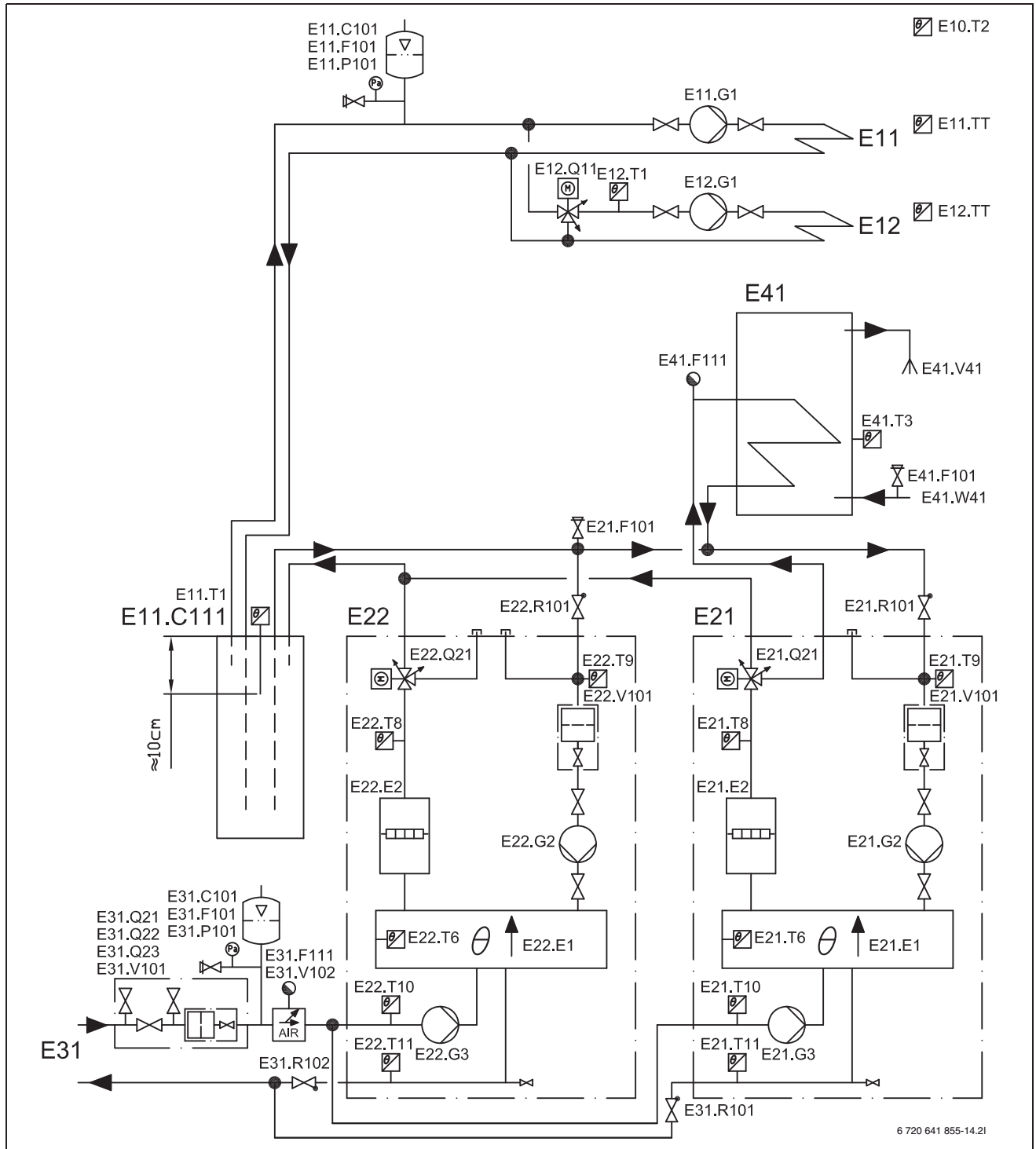
Kuva 62 Kaksi lämpöpumpua (kaskadikytkentä), joissa shunttaamaton ja shuntattu lämmityspiiri, työväli ja ulkoinen käyttöveden lämmitys
