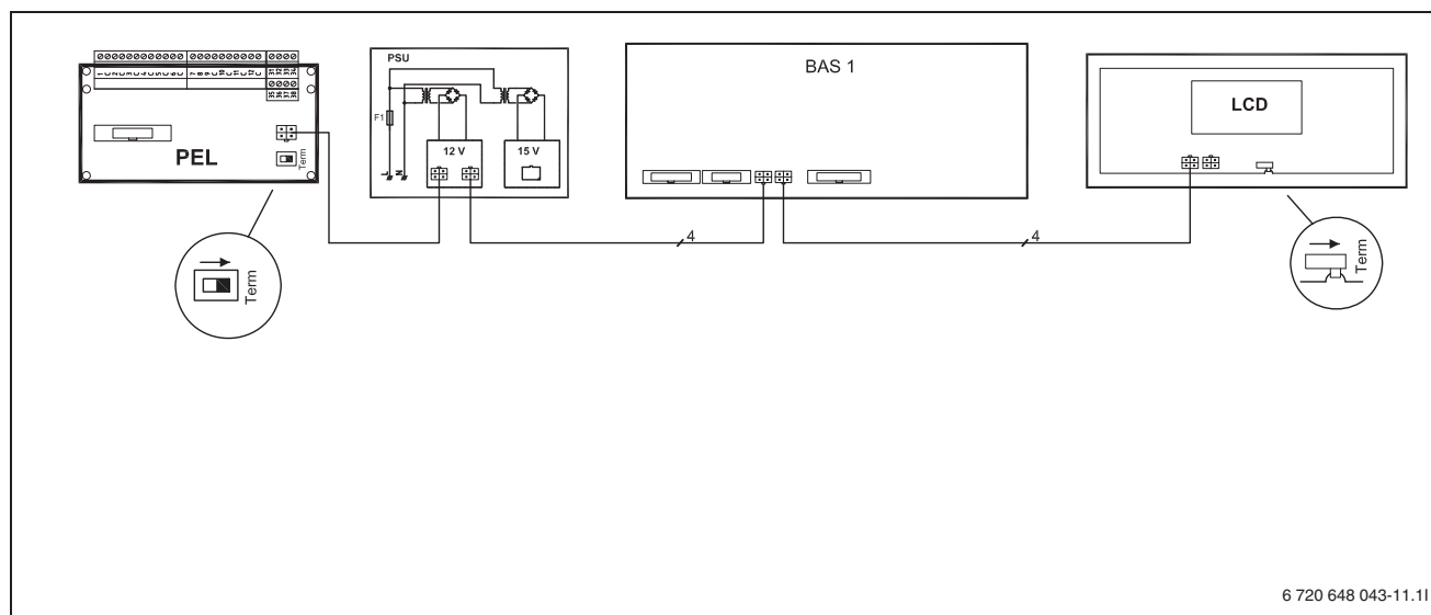
Kuva 39 CANBus, yleiskatsaus
