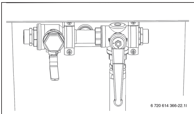
Kuva 26 Täyttöasema sekoitustilassa
