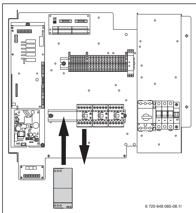
Kuva 33 Korvaa kontaktori
