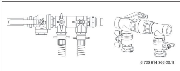
Kuva 28 Täyttösarjat paineennostoasennossa
