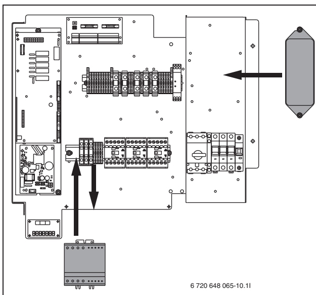
Kuva 36 Pehmökäynnistyksen ja EMC-suodattimen asennus
