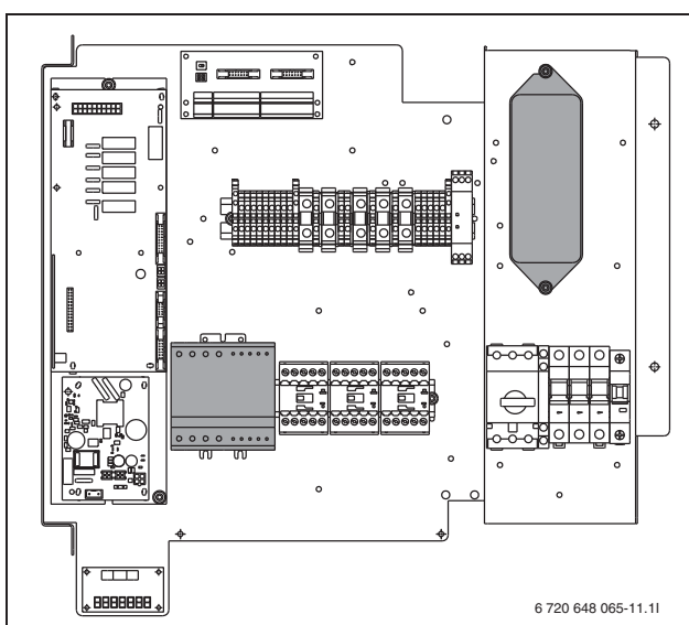
Kuva 37 Asenna pehmökäynnistys ja suodatin.
