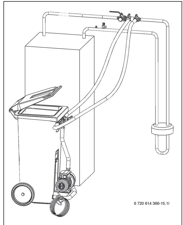
Kuva 24 Täyttö täyttöasemalla
