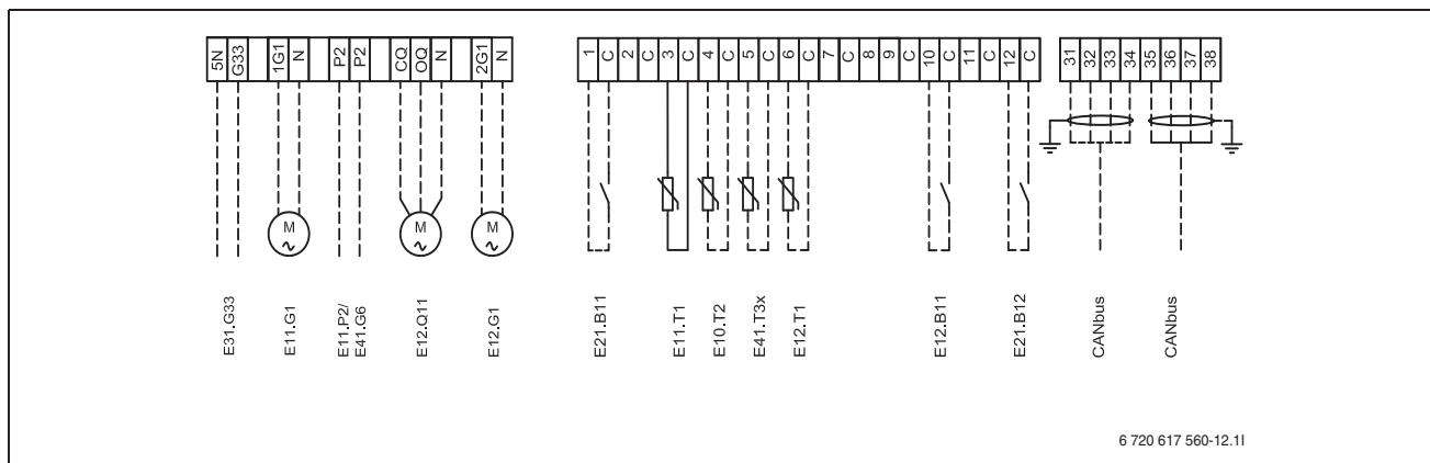
Kuva 44 Ulkoiset liitännät
