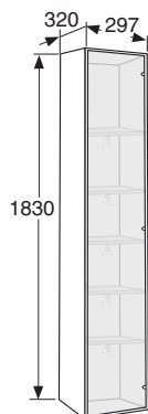
Korkea kaappi ovella/ Högsåp med dörr 297 mm
