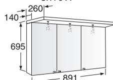
Peilikaappi halogeenirampilla/ Spegelskåp med halogenramp 891 mm 3x10W
