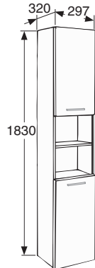
Korkea kaappi avohyllyllä/ Högsåp med öppen hylla 297 mm
