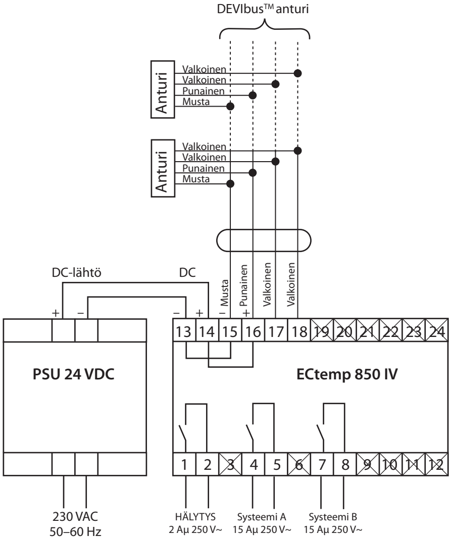
Kuva A — Kytentäkaavio DEVireg™ 850 IV
