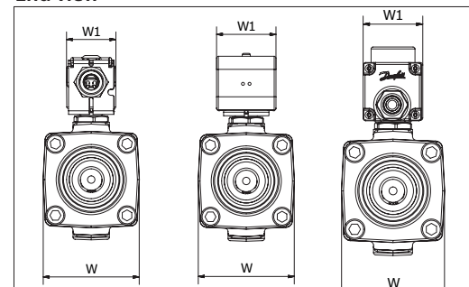
Conduit hub 1)
