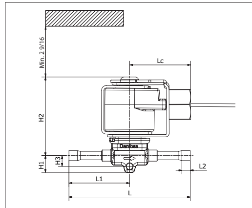
Terminal box 3)
