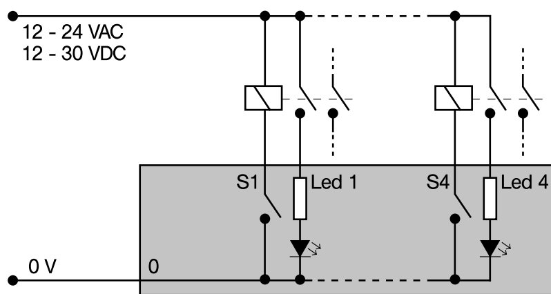
KytKentä sysäysreleille.
