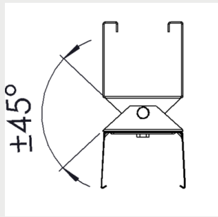
Säädettyä valaisinkiskokannake
