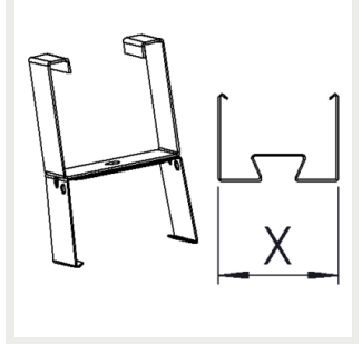
3508172 Gamma Eco S ripustuskiskokannake 82 (7)
