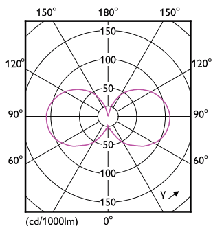
LEDLuster MAS SLR P45 2,5W E14 927 CL-LDD
