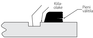
Putki syvällä urilla – kuva 1 Ylikorostettu selvyyden vuoksi
