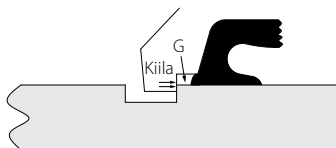
Alimittainen putki/yhde
