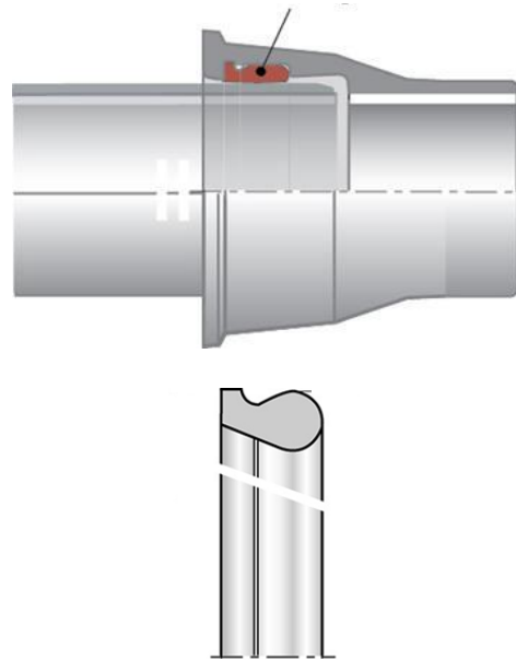
Tyton tiiviste
