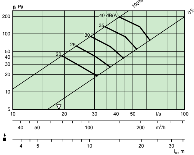
ALG 200 x 100 + TRG-B Ø125, Tuloilma
