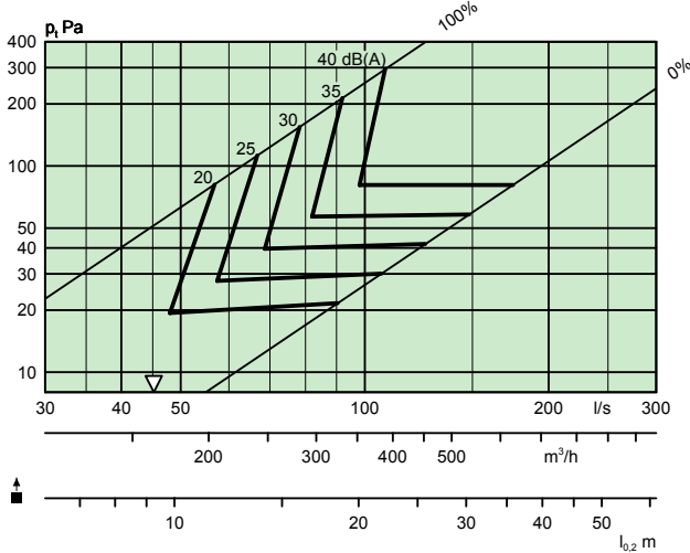
ALG 400 x 150 + TRG-B Ø250, Tuloilma
