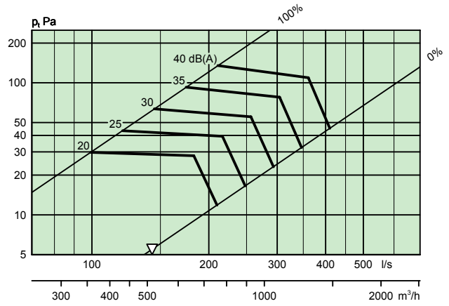
ALG 600 x 200 + TRG-B Ø315, Poistoilma
