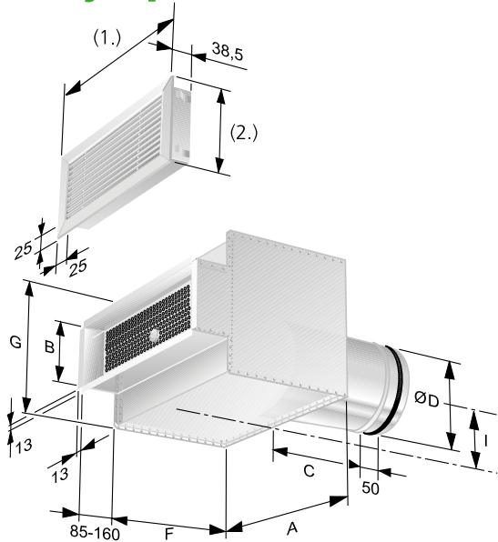
Kuva 2. ALG/TRG. (1.) Nimellislevyys + 30 mm (2.) Nim. kork. + 30 mm Säleikön tarkat mitat saadaan lisäämällä nimellismittoihin kuvan ALG mukaiset mitat. Aukontekomitta = nimellismitta (säleikön kokomerkinä).
