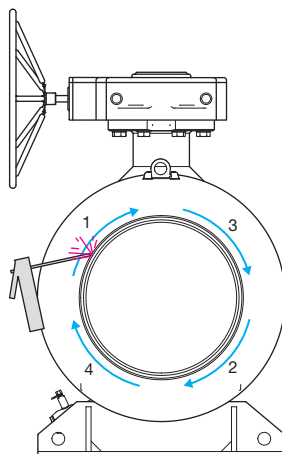
Kuva 6. Saumojen hitsaus.
