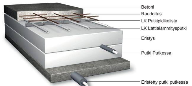
Putki putkessa -rakenteen asennus betonilaattaan, jossa on lattialämmitys.
