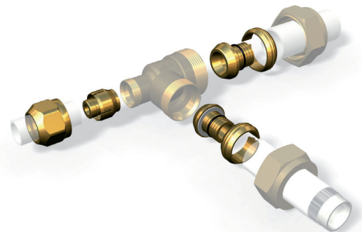
Esimerkki PE-X- ja PAL-putken liittämisestä LK Liitinsarjalla.
