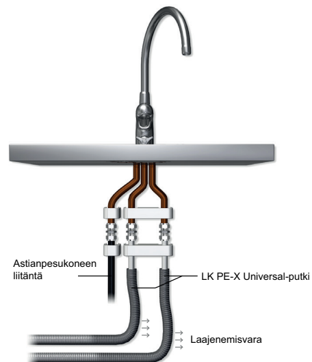
Esimerkkiasennus kuparisilla liitosputkilla varustetun keittiösekoittajan asennuksesta putki putkessa -rakenteisen LK PE-X- ja PAL Universal-putken kanssa.
