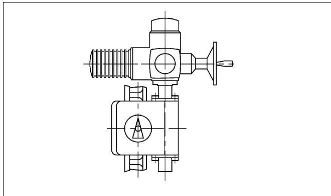
Kuva 30 Sähkökäyttö
