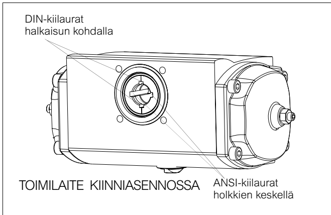
Fig. 22. Toimilaitteen kiilaurien asennot
