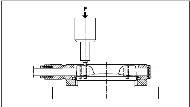
Kuva 17 Sokkien puristaminen
