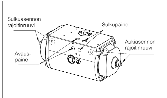
Fig. 23. Toimilaitteen liitännät
