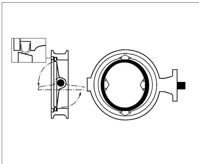
Kuva 1 Venttiilin toimintaperiaate
