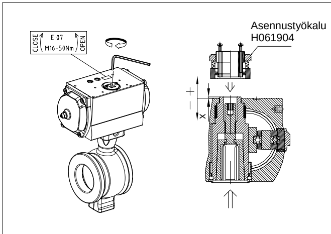
Kuva 21 Väliholkin kiristys
