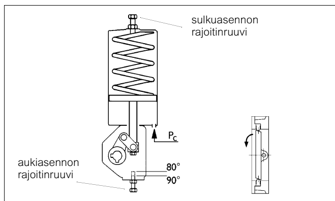
Kuva 27 Sylinteritoimilaite, sarja B1JA
