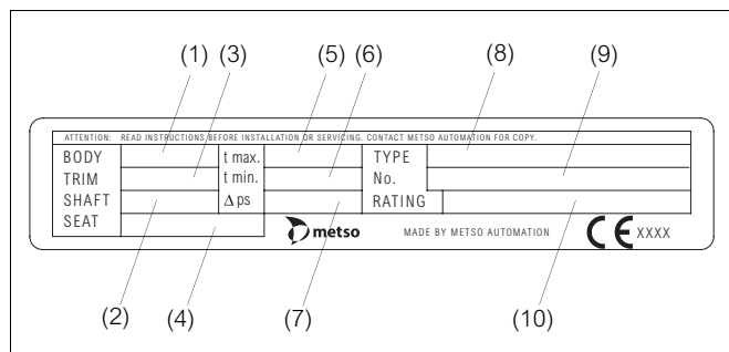
Kuva 2 Konekilpi
