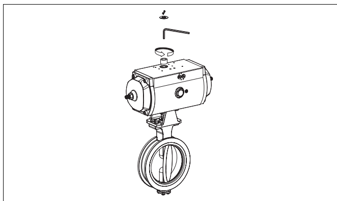
Fig. 18. EC/EJ-toimilaitteen irrottaminen
