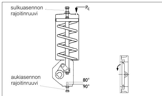
Kuva 26 Sylinteritoimilaite, sarja B1J
