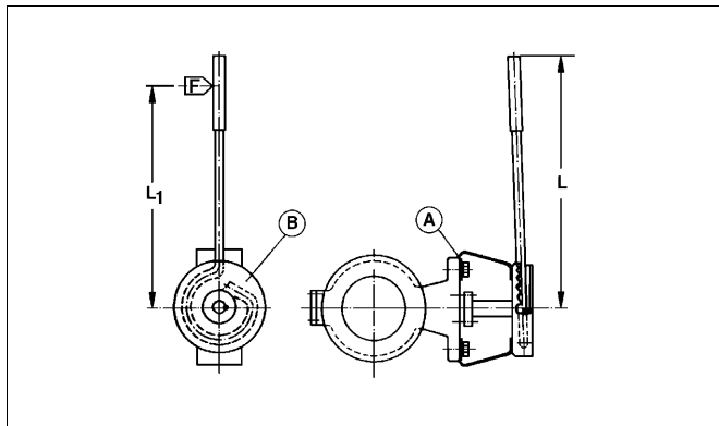
Kuva 29 Käsivipu, sarja RH
