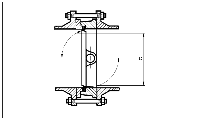
Kuva 6 Asennusmitat
