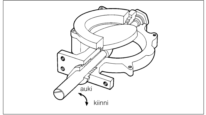
Kuva 13 Lämpän ja tiivisteen keskinäinen asento
