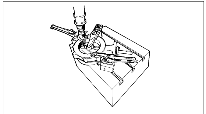
Kuva 14 Sokkien poraaminen
