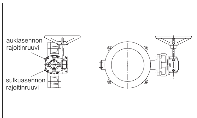
Kuva 28 Käsikäyttö, sarja M
