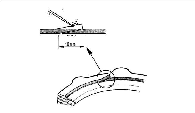
Kuva 12 Tiivistenauhan asennus
