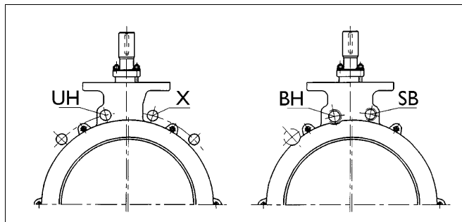
Kuva 7 Asennusvaihtoehdot
