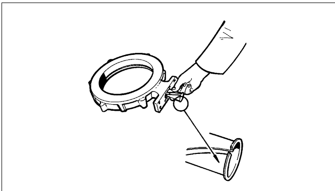
Kuva 16 Vakiolaakerien asennus
