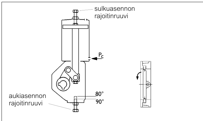
Kuva 25 Sylinteritoimilaite, sarja B1C
