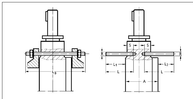
Kuva 8 Ruuvien asennusmitat, asennusvaihtoehto SB
