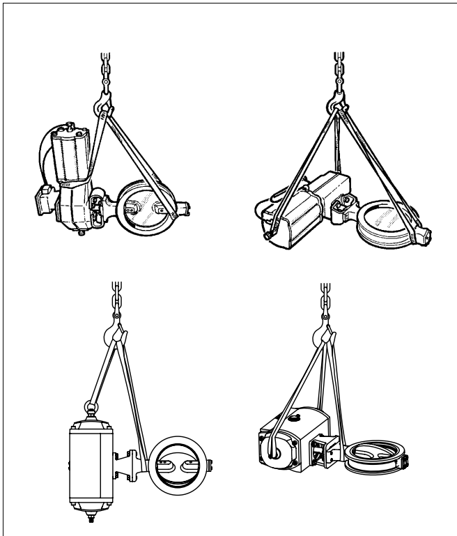
Kuva 3 Venttiilin nostaminen
