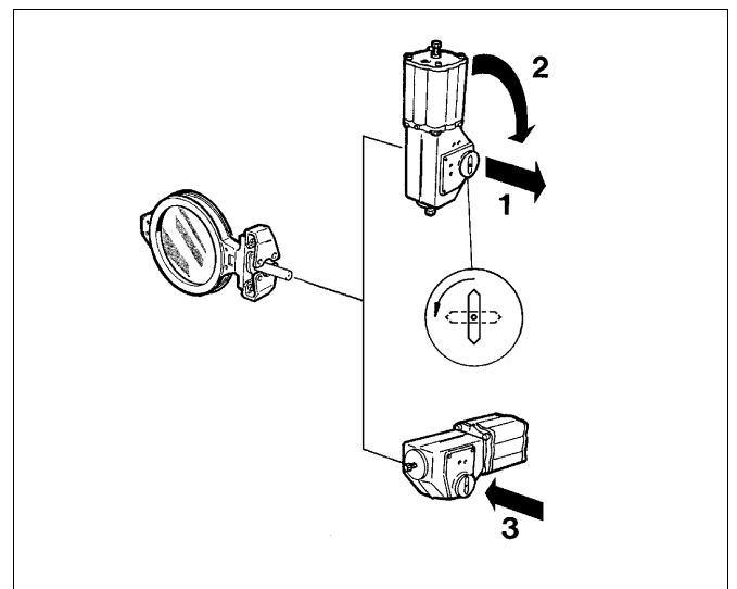
Kuva 24 Asennusasennon vaihto
