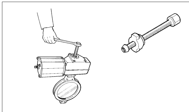
Kuva 19 B-sarjan toimilaitteen irrottaminen ulosvetäjällä
