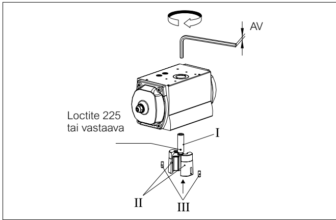
Fig. 20. Väliholkin asennus
