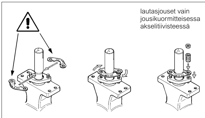
Kuva 10 Pidätinlevyjen asennus
