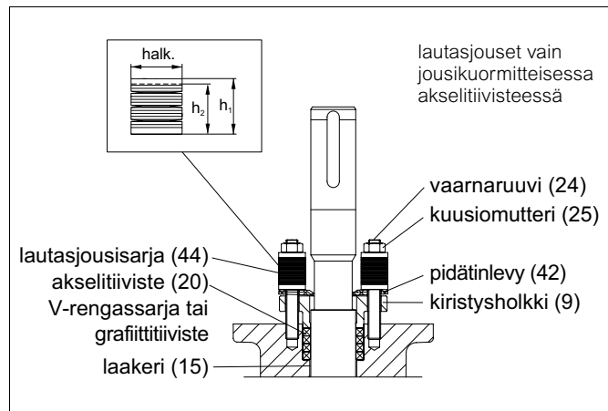
Fig. 11. Akselitiiviste
