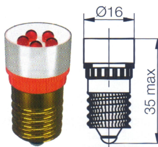
Socket E14
