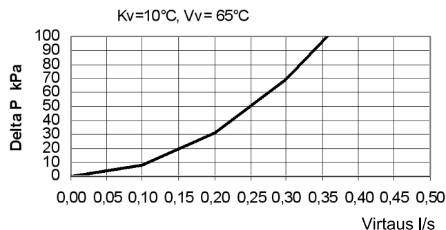
Painehäviökäyrä
