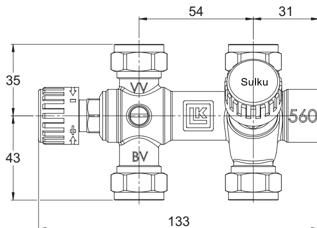
Mittapiirros
