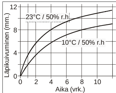
Kaavio 1: Sikaflex®-221:n kuivumisnopeus
