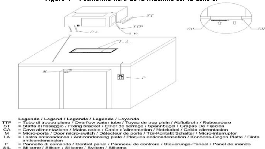
Figure 4 – Positionnement de la machine sur la cellule.
