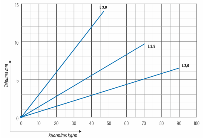
KRA/KRB 40 | LEVEYDET 400, 500, 600
