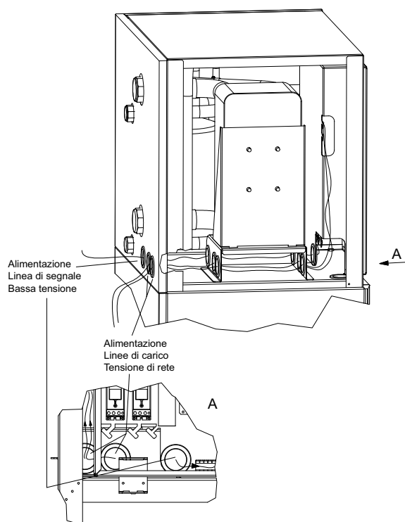
Fig. 7.4: Ingresso cavi quadro di comando
