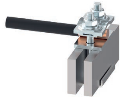
KL800 asennus
