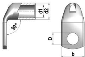
90° -kulmakaapelikengät
