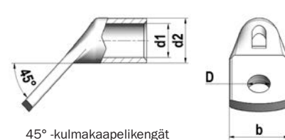
45° -kulmakaapelikengät
