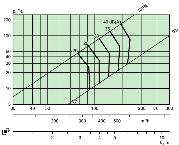
LOCKZONE C 315-500+ALS 250-315 – Yksi mittamuutos
