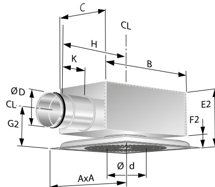
Kuva 7. LOCKZONE Ceiling ja ALS. Matala rakennekorkeus
