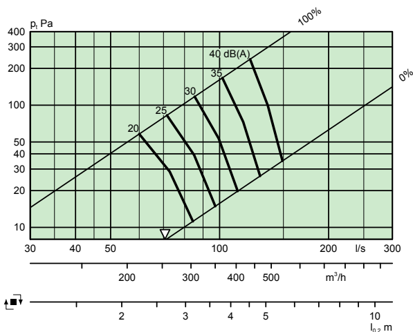
LOCKZONE C 315-500+ALS 200-315 – Kaksi mittamuutosta
