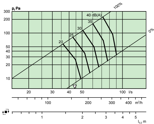
LOCKZONE C 200-500 + ALS 160-200 – Yksi mittamuutos
