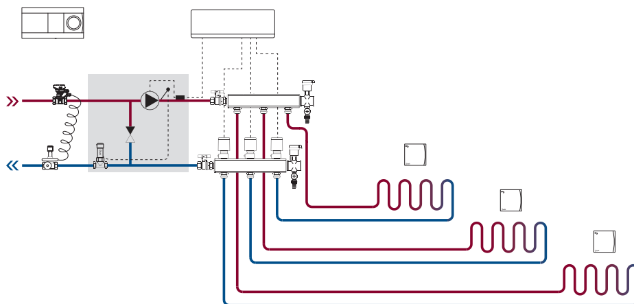
Esimerkki 2: 2-putkijärjestelmä ja sekoitusventtiili (valinnainen syöttölämpötilan ohjaus)
