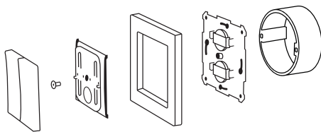
Asennus kojerasiaan ruuvilla.
