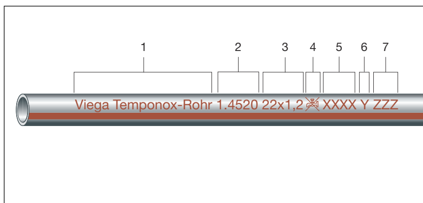
Fig. 6: Temponox pipe 1.4520
