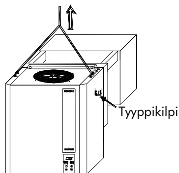
Kuva 2 – Laitteen nostaminen.
