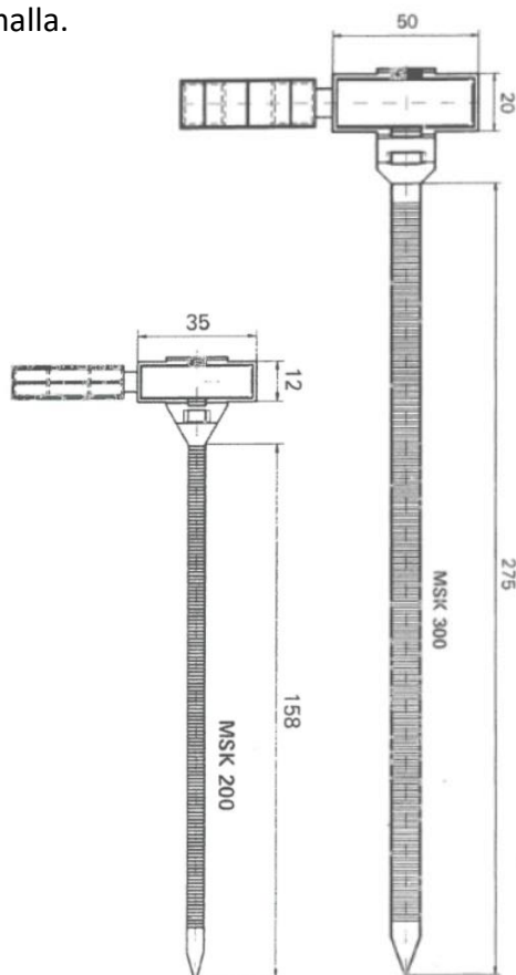
Kuva 2. MSK300-merkintäpanta
