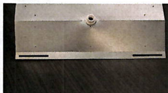
2. Montera röranslutningen i avsett uttag
