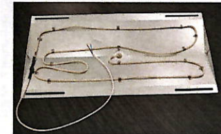
3. Insira o cabo de aquecimento e ligue-o usando os suportes de montagem pré-montados.
