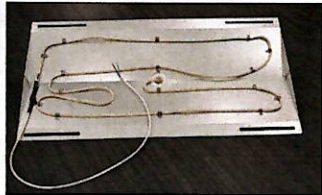
3. Aseta lämmityskaapeli paikalleen ja kiinnitä se valmiiksi kootuilla kiinnikkeillä.
