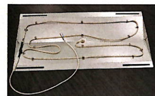
3. Inserire il cavo riscaldante e fissarlo usando le staffe di montaggio preassemblate.
