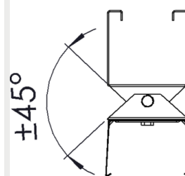
Säädettävä valaisinkiskokannake
