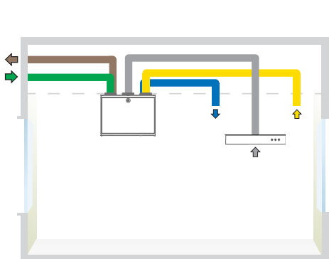
CASA W4 Smart xs L kanavaliitännät ja liesikupu liitettynä ilmanvaihtoon keittiökanavayhteeseen.
