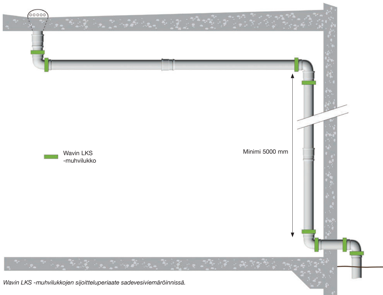
Wavin LKS -muhvilukon asennus.
