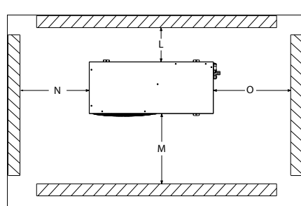
Bild 1: Mindestmontageabstände
