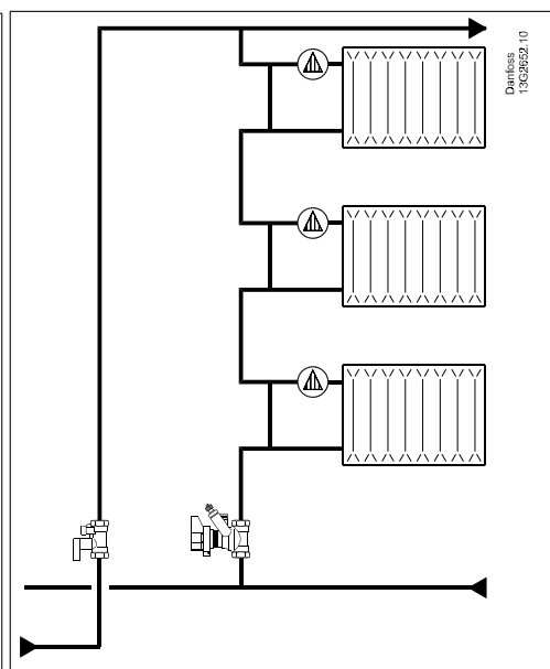
1-putkinen järjestelmä
