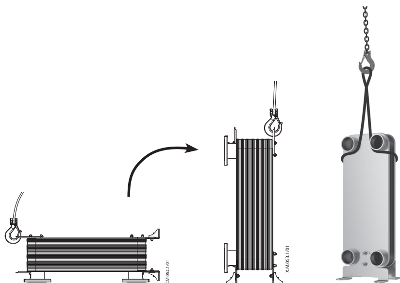
Fig. 2 Løft / Fig. 2 Lifting / Abb. 2 Heben / Fig. 2 Levage / Fig. 2 Elevación / Fig. 2 Sollevamento / Fig. 2 Lyftning / Fig. 2 Hysen / Kuva 2 Nostaminen / 2 pav. Kėlimas / 2. att. Pacēšana / Joonis 2 Tõstmine / Obr. 2 Zdvíhanie / Slika 2 Dviganje / Sl. 2 Podizanje / 图 2 起吊 / Фуз. 2 Повдигане / Slika 2 Podizanje / Fig. 2 Ridicare / 2. ábra: Emelés / Obr. 2 Zvedání / Rys. 2 Podnoszenie / Рис. 2 Подъем
