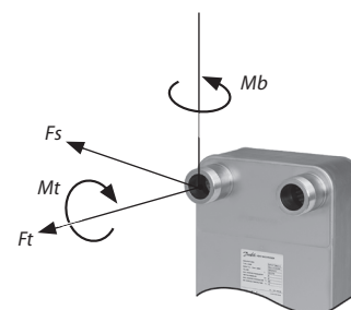
Fig. 3 Drejningsmoment / Fig. 3 Torque force / Abb. 3 Drehmoment / Fig. 3 Force de couple / Fig. 3 Esfuerzo de torsión / Fig. 3 Forza coppia / Fig. 3 Vridmoment / Fig. 3 Torsiekracht / Kuva 3 Vääntävä voima / 3 pav. Sukimo momento jėga / 3. att. Griezes momenta spēks / Joonis 3 Pöördemomendi tugevus / Obr. 3 Síla krútiaceho momentu / Slika 3 Navorna síla / Sl. 3 Síla okretnog momenta / 图 3 扭力 / Фуз. 3 Въртящ момент / Slika 3 Síla obrtnog momenta / Fig. 3 Força de cuplului / 3. ábra: Azonosító címke / Obr. 3 Kruptivá síla / Rys. 3 Síla momentu obrotowego / Рис. 3 Напряжения, действующие на патрубки
