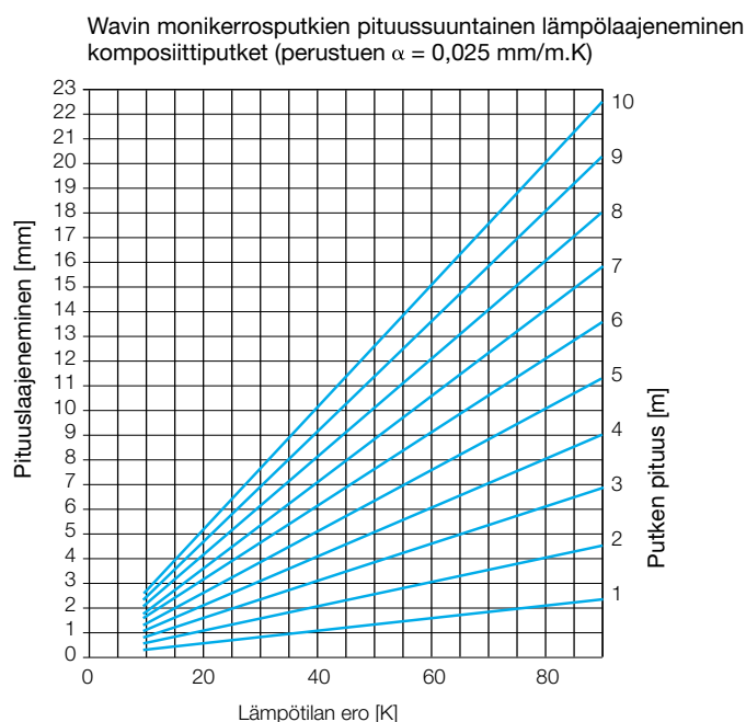
Kuva 36: Pituussuuntainen lämpölaajeneminen.
