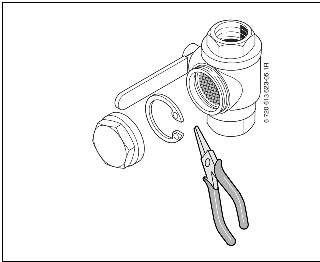
Kuva 31 Lukkorenkaalla varustettu suodatinvaihtoehto
