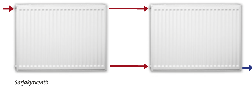
Ristikkäinen kytkentä
