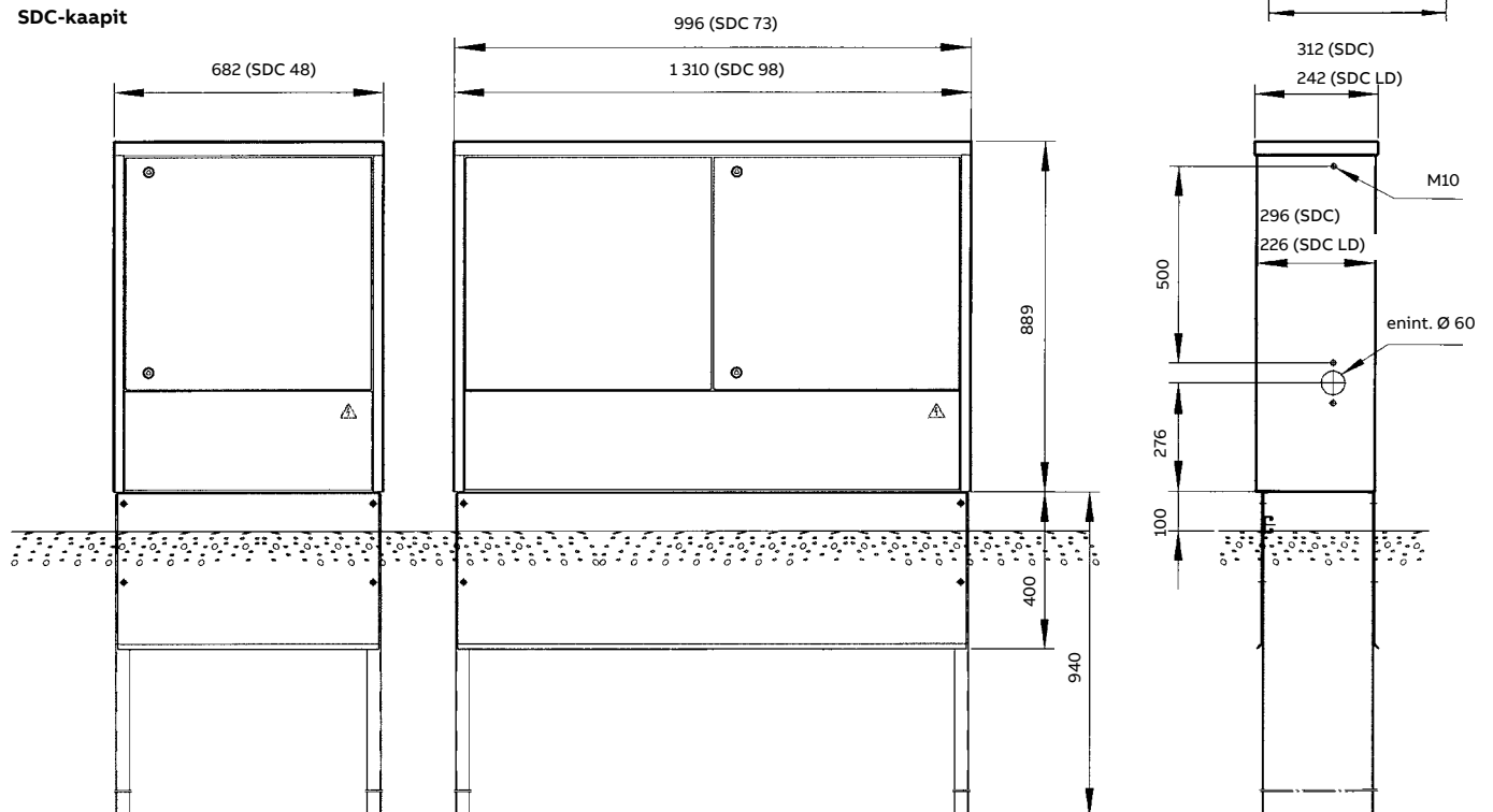
SDC-kaapit
