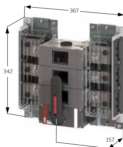
LBOD 800
