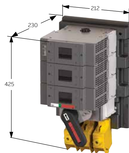
SEKOD 355
