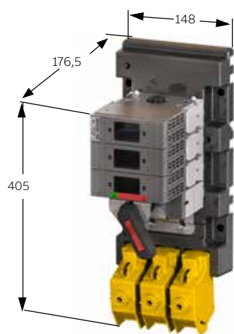
SEKOD 125
