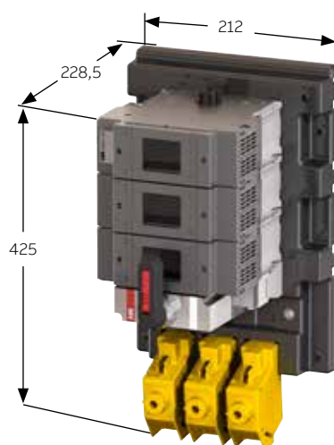
SEKOD 224
