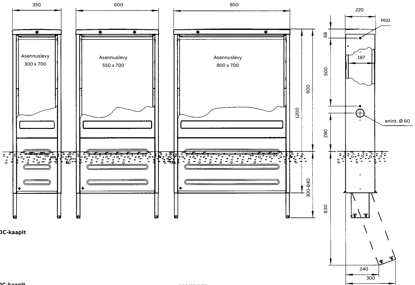
SDC-kaapit
