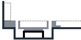
Poikkileikkaus lattiakaivokalusteesta, jossa on kehys/ Cassette-ratkaisu harjattua terästä.
