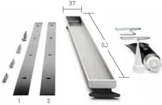
Korotussarja: K: 1 ja 2 mm. Säädä Cassetten korkeutta. Korotuspalat asennetaan Cassetten ja rungon väliin.
