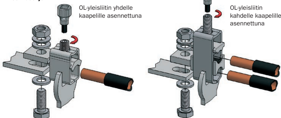
OL 6-70MZ / OL 70-185Z / OL 185-300Z
