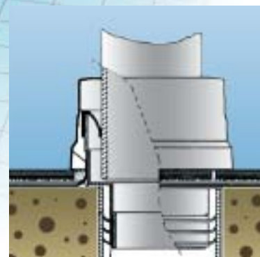
Laatta-asennus
